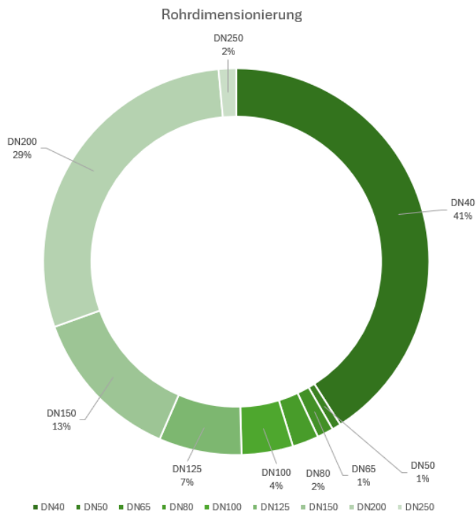
Abbildung 19: Rohrdimensionierungen und Verteilung eines 10°C Uferfiltrationsnetzes (Quelle: eigene Darstellung nach SO Ing.)
